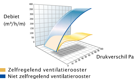
Luchtdebiet onafhankelijk van de wind
