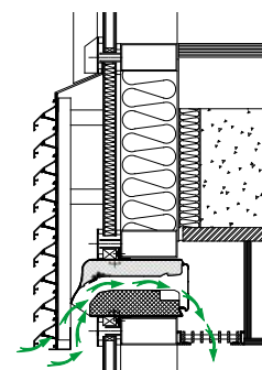
Verborg installatie (achter lamellen)
