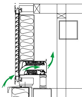
Verborg installatie (achter lamellen)
