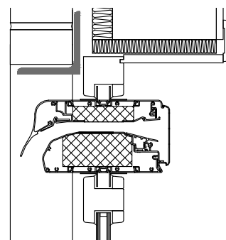
Tussen profielen (traverse) (aanbevolen installatiewijze)
